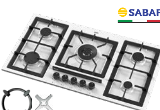
E518W پلوپز وسط (بدنه لعابی سفید) Size: 91 x 51 cm Cutting: 880 x 480 mm
