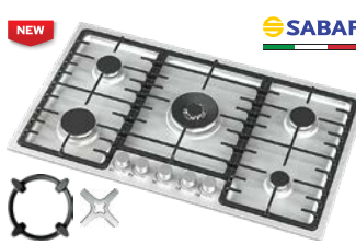
S508 پلوپز وسط Size: 90 x 52 cm Cutting: 875 x 495 mm
