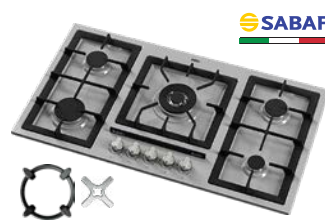
E518C پلوپز وسط (بدنه لعابی طوسی) Size: 91 x 51 cm Cutting: 880 x 480 mm
