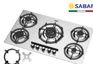
S506 پلوپز وسط Size: 90 x 52 cm Cutting: 880 x 495 mm
